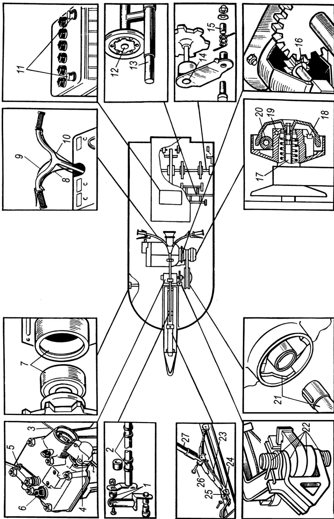
Рисунок 23— Схема смазки
