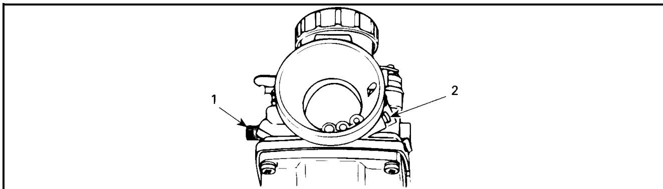
Рисунок 25 – Регулировка карбюратора MIKUNI VM34-619
