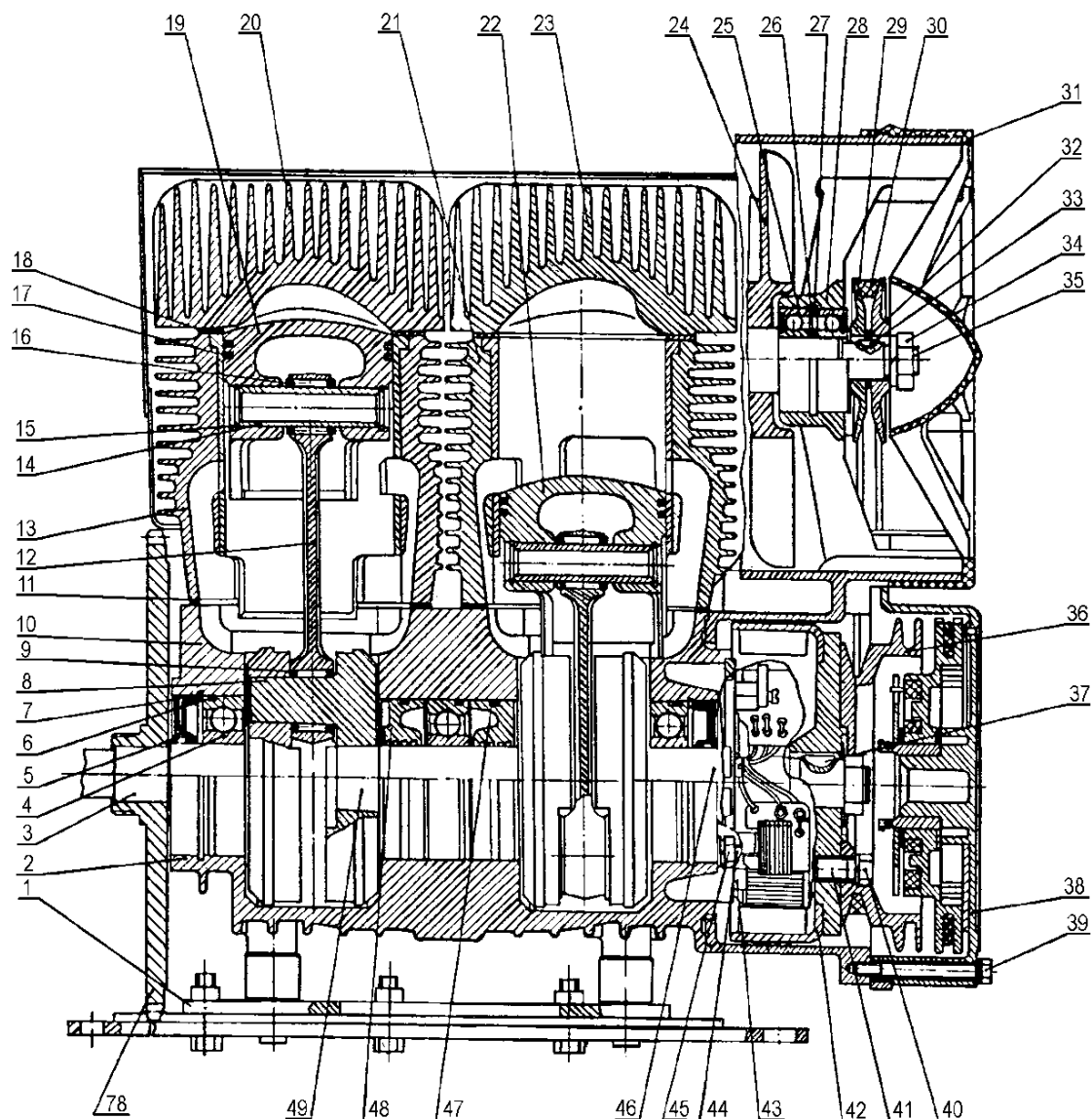
Рисунок 3 – Двигатель
