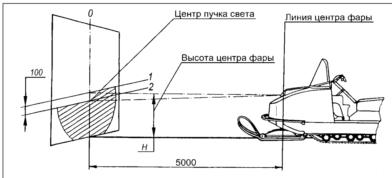
Рисунок 30 – Регулировка фары
