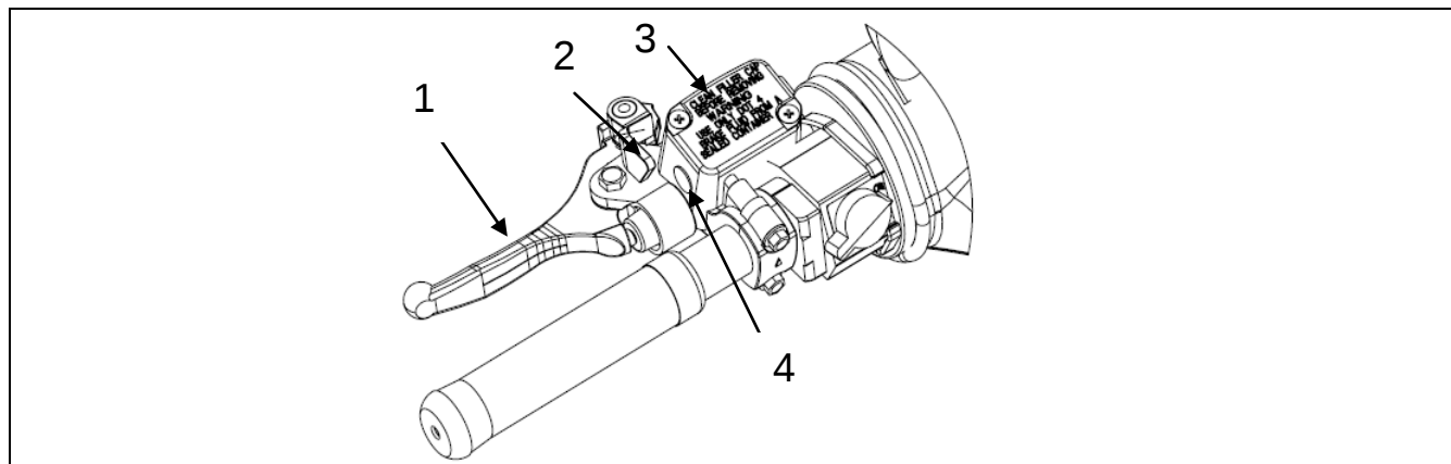
Рисунок 17 – Расположение гидравлической тормозной системы и фиксатора стояночного тормоза
