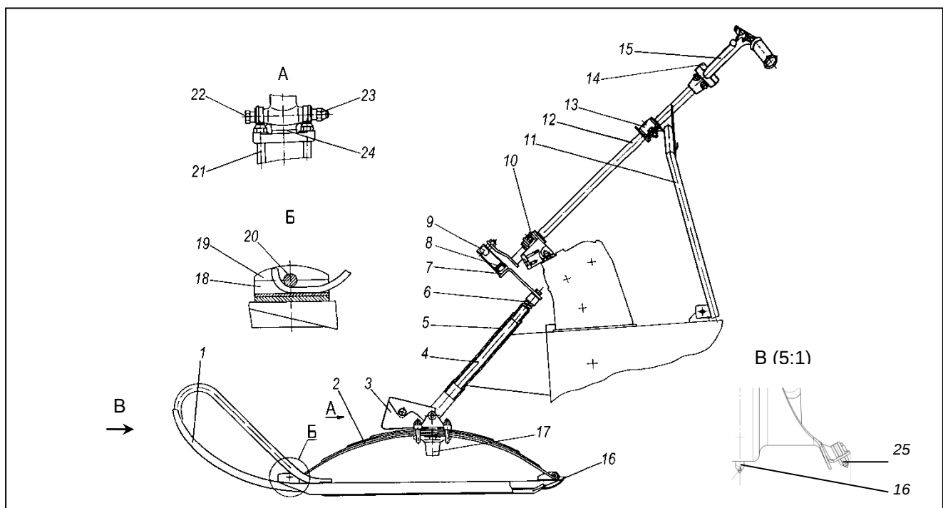
Рисунок 11 – Рулевое управление
