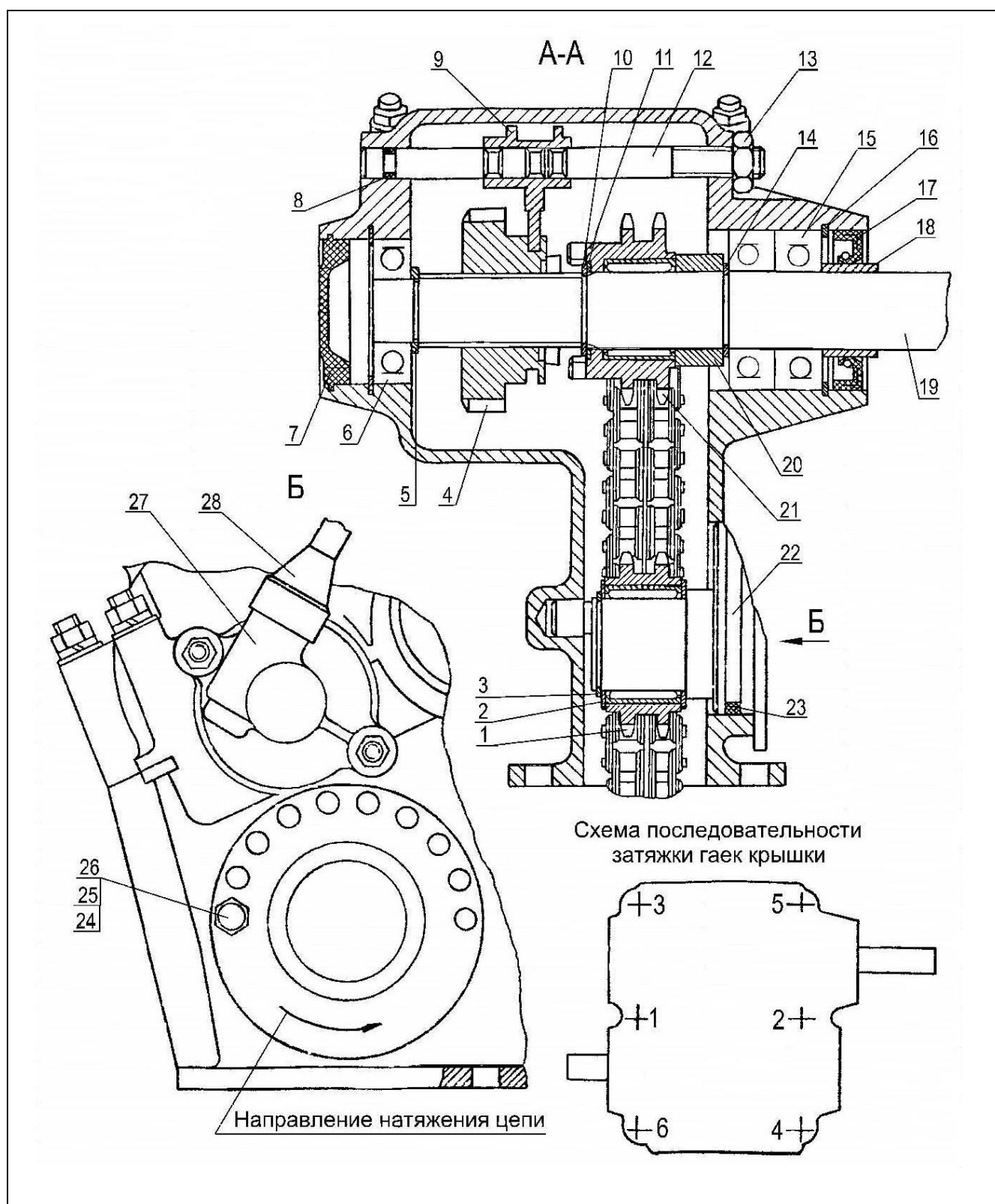
Рисунок 7 – Коробка реверса БУРАН А, АД
