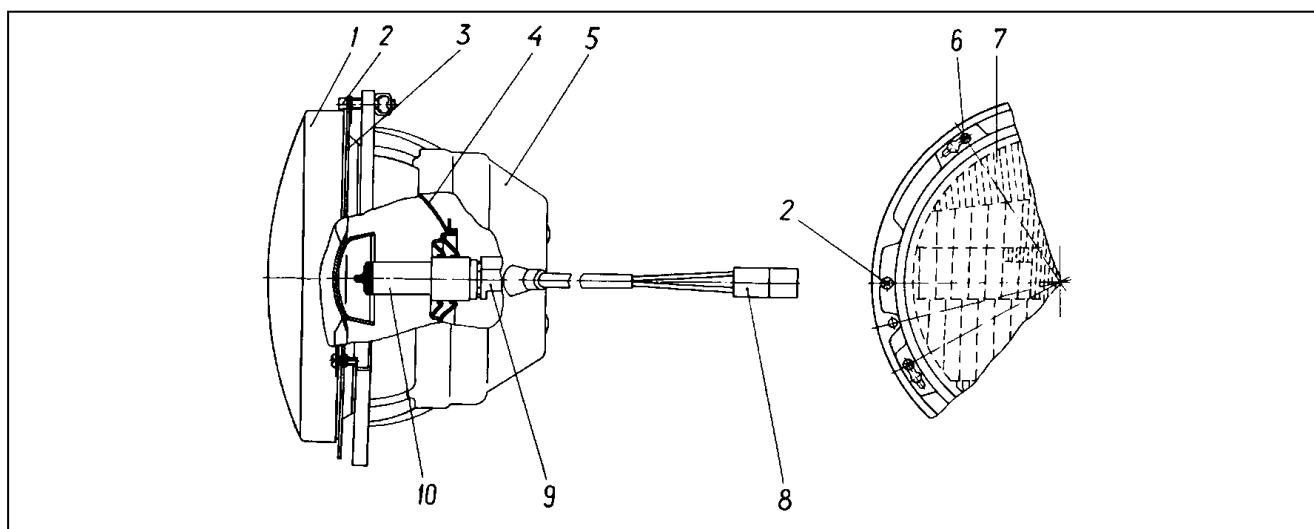
Рисунок 20 – Фара
